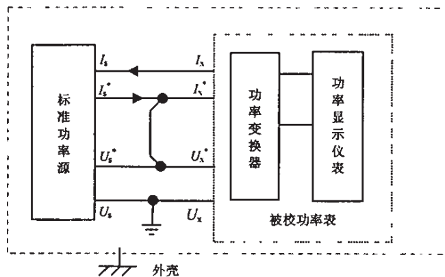
图 2 标准功率源法校准功率表的原理接线图
