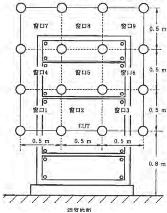
图 J.1 A 台式设备将校准区域划分为数个 0.5 m x 0.5 m 窗口的实例
