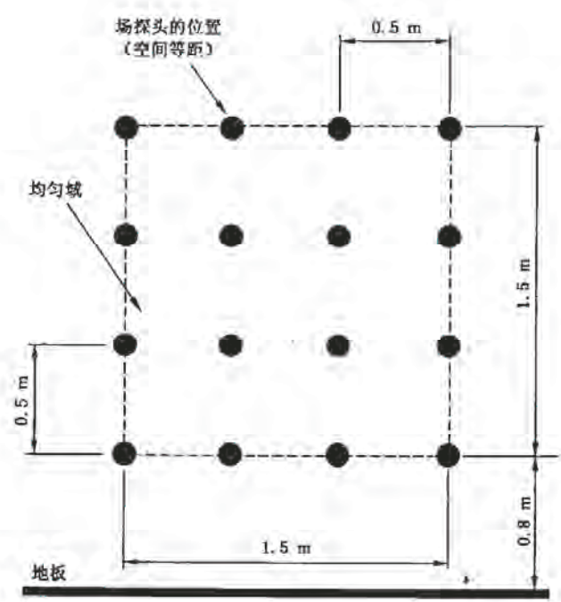
图 4 场校准,均匀域的尺寸
