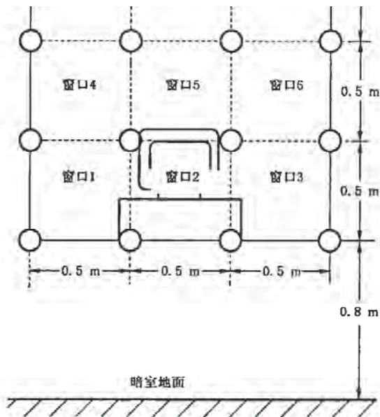
图 J.1 A 台式设备将校准区域划分为数个 0.5 m x 0.5 m 窗口的实例
